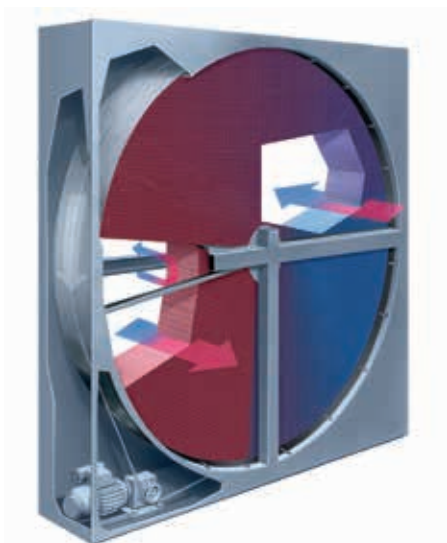
Wärmerad mit hohem Wirkungsgrad von 80 % als effiziente Methode zur Wärmerückgewinnung.
